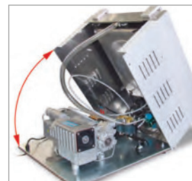
Ouverture frontale de la machine permettant d'accéder à l'intérieur pour faciliter le service technique.
